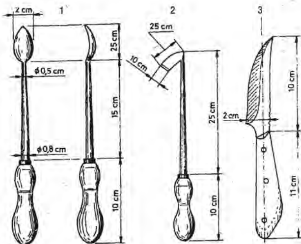
1. ábra. A preparálás szerszámai. 1. kaparókanál, 2. kaparóhorog, 3. nyúzókés
